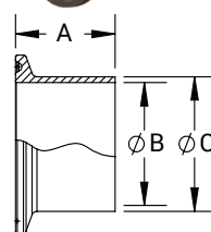
BPE Table DT-4.1.4-1 ASME BPE 2019
