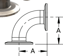
BPE Table DT-4.1.1-3 ASME BPE 2019
